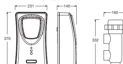
Dimensiones (mm)
