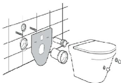
Antiacústico para inodoro y bide Suspendido
